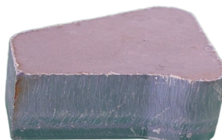
30mm碳钢混气切割效果
